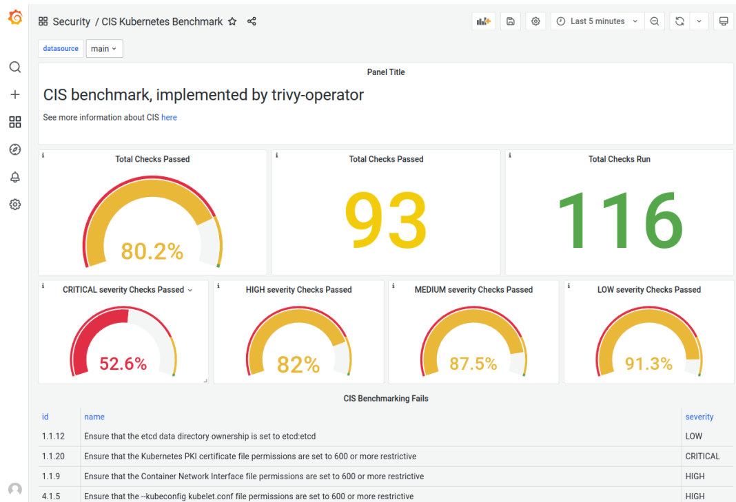
Рисунок 2. Пример дашборда CIS Kubernetes Benchmark.
