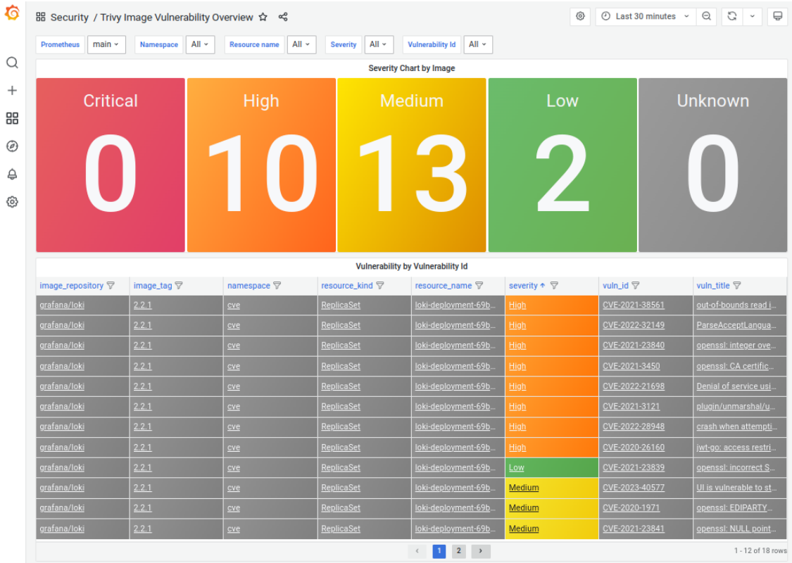
Рисунок 5. Пример дашборда Trivy Image Vulnerability Overview.
